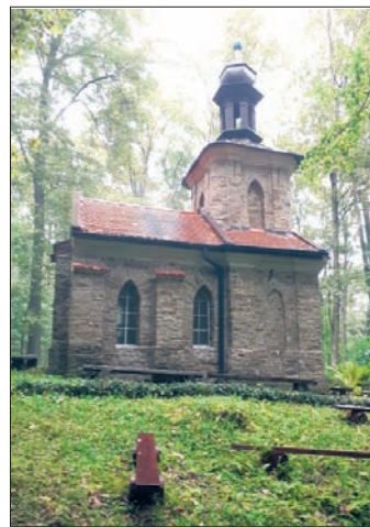
Kapliczka konfederatów na górze Jasień w Suchej Beskidzkiej
