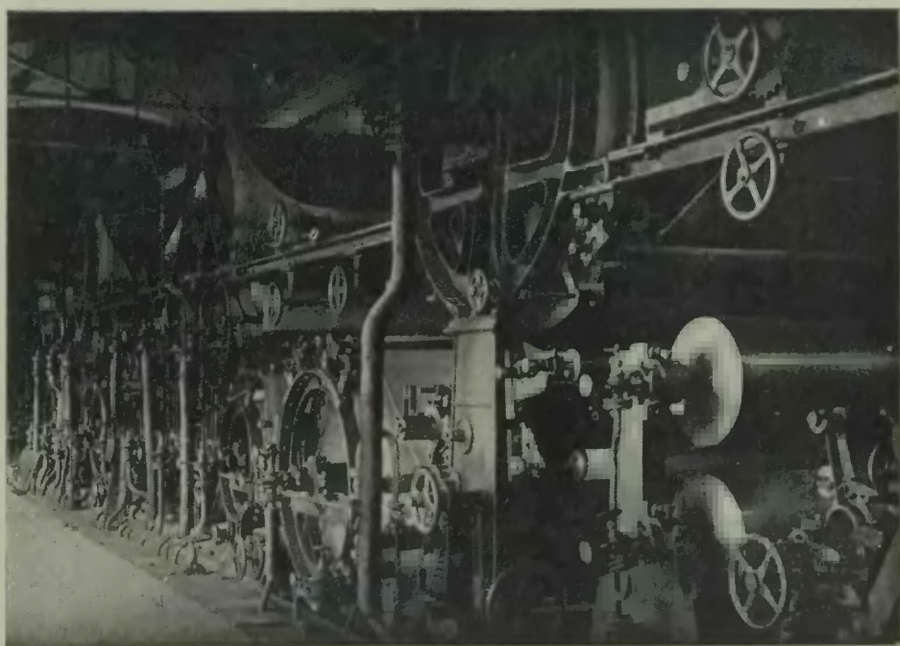
Papierfabrik Mirkow, Pergamentiermaschinen
