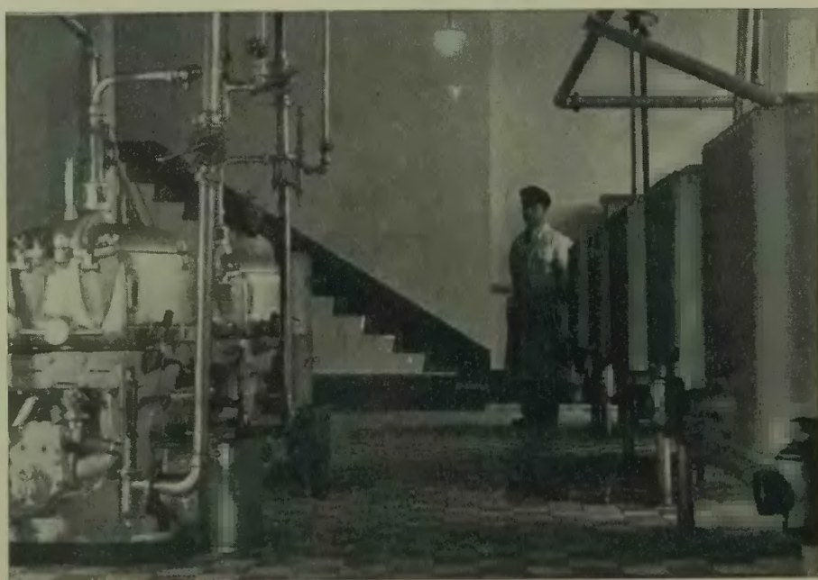
Butterschmelzanlage
