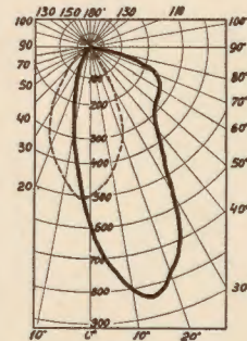
Wykres rozsyłu strumienia świetlnego przy użyciu żarówki 100 W o wydajności 1000 lumenów. — w kierunku A - - " " B
