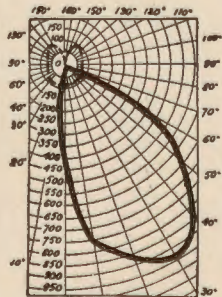
Wykres rozsyłu strumienia świetlnego przy użyciu żarówki 100 W o wydajności 1000 lumenów, dla opraw Nr. 36565-6.
