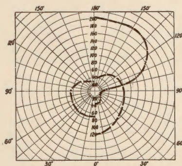
Wykres rozsyłu strumienia świetlnego dla źródła światła o wydajności 1000 lum. — dla opraw Nr. 36953, 36955, 36963 — dla opraw Nr. 34113, 34115
