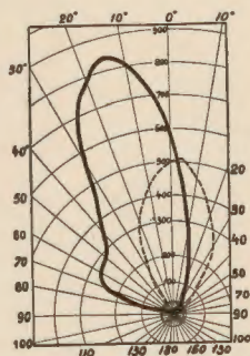
Wykres rozsyłu strumienia świetlnego przy użyciu żarówki 100 W o wydajności 1000 lumenów. — w kierunku A - - " " B
