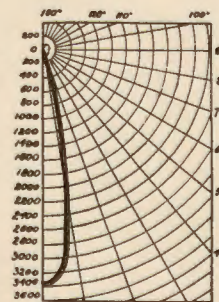
Wykres rozsyłu strumienia świetlnego przy użyciu żarówki 100 W o wydajności 1000 lumenów, dla opraw Nr. 36567-8.
