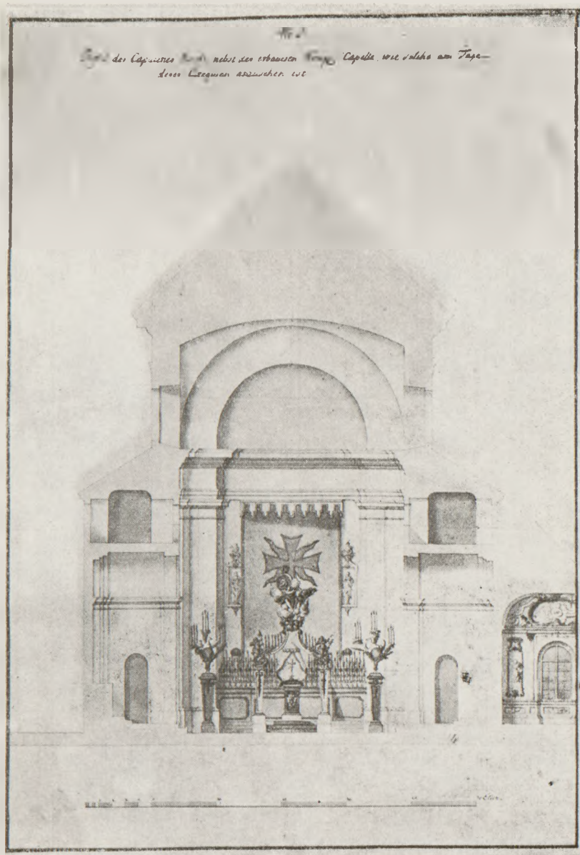
Kościół OO. Kapucynów. Przekrój poprzeczny z kaplicą królewską z widokiem dekoracji żałobnej (nr kat. 306)
