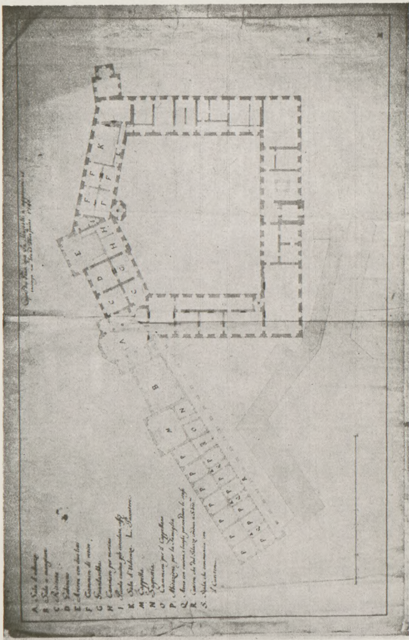
Zamek Królewski Rzut pierwszego piętra (nr kat. 171)
