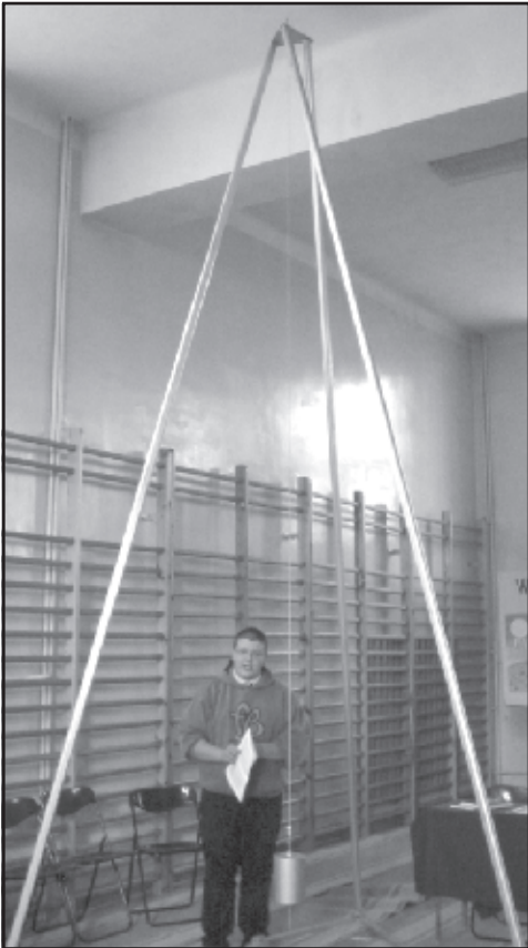
Wahadło Foucaulta.
