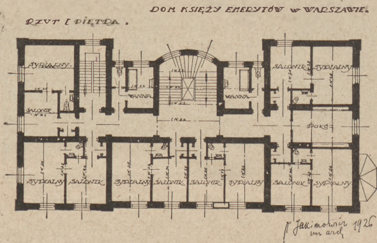
Plan domu Księżych Emerytów.
