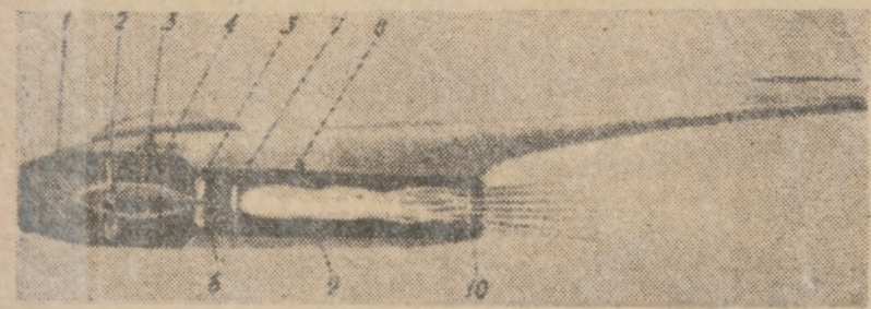
Schematyczny przekrój modelu samolotu odrzutowego z silnikiem sprężarkowym: 1) stożek czołowy, 2) czterokierunkowa śruba, 3) łącząca powłoka, 4) motorek, 5) rurka doprowadzająca paliwo do zbiorniczka, 6) mieszalnik, 7) rurka do wtrysku paliwa, 8) rozpryskiwacz paliwa, 9) elektryczna świeca, 10) rurka wylotowa gazów odrzutowych.
