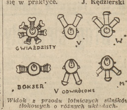
Widok z przodu lotniczych silników tłokowych o różnych układach.
