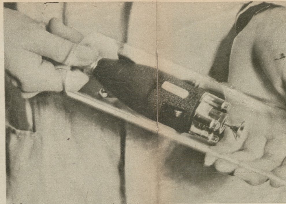
Mikro-nadajnik — telewizyjny szlagier tegorocznych targów w Hanowerze. Pomaga — w wykrywaniu — uszkodzeń przewodów podziemnych. Dzięki swym wymiarom aparat mieści się np. nawet w 1,5 cm rurze gazowej, skąd przekazuje obraz uszkodzonego przewodu. Zdalnie kierowany przesuwa się wzdłuż rury w żądanym kierunku. CAF
