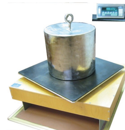
Stanowiska pomiarowe do przekazywania jednostki masy od 50 kg do 500 kg i 1000 kg w klasie F_2
