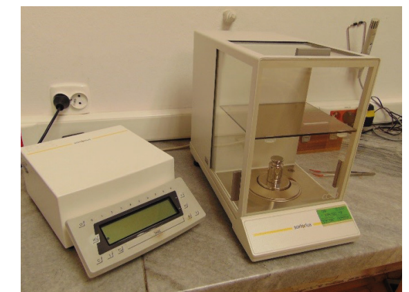
Stanowiska do przekazywania jednostki masy od 200 g do 1 g
