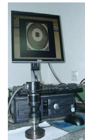
Stanowiska wzorca odniesienia twardości Brinella wraz z mikroskopem
