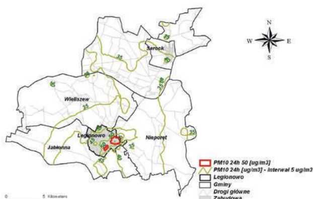
Rysunek 3.57 Rozkład stężeń pyłu zawieszonego PM 10 o okresie uśredniania wyników pomiarów 24 godzin, powodowanych emisją całkowitą, w powiecie legionowskim w 2006 roku
