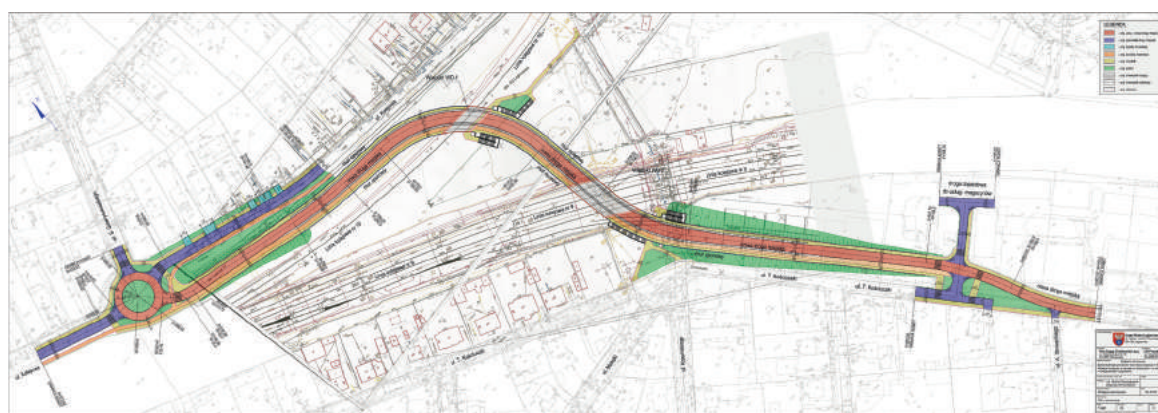
▲ Projekt pierwszej przeprawy w ul. Krasińskiego
