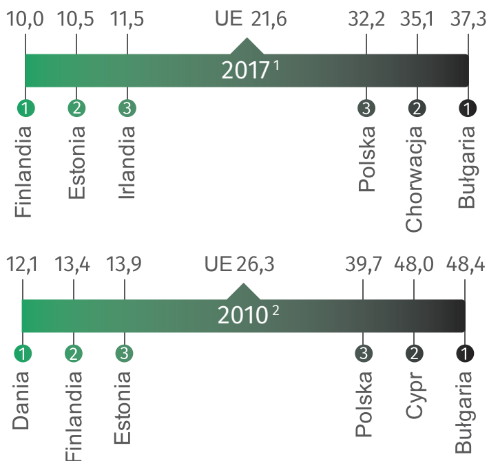
PM10 (mikrogramy na m 3 )
