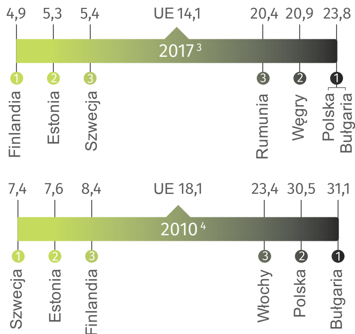
PM 2,5 (mikrogramy na m 3 )
