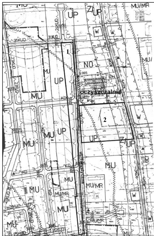
Fragment z rysunku Miejscowego Planu Zagospodarowania Przestrzennego - 2004 r. Legenda: UP - tereny usługowo - produkcyjne, MU - tereny mieszkaniowo - usługowe, 1 - działka Nr 426 zakupiona przez firmę Hetman w 2011 r., 2 - tereny, na których funkcjonuje firma Hetman, gdzie prowadzona będzie modernizacja.
