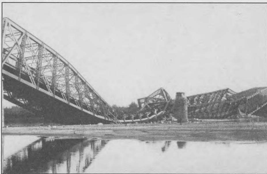
Fotografia zniszczonego mostu M. Marszewskiego w Zegrzu, 1915 r.
