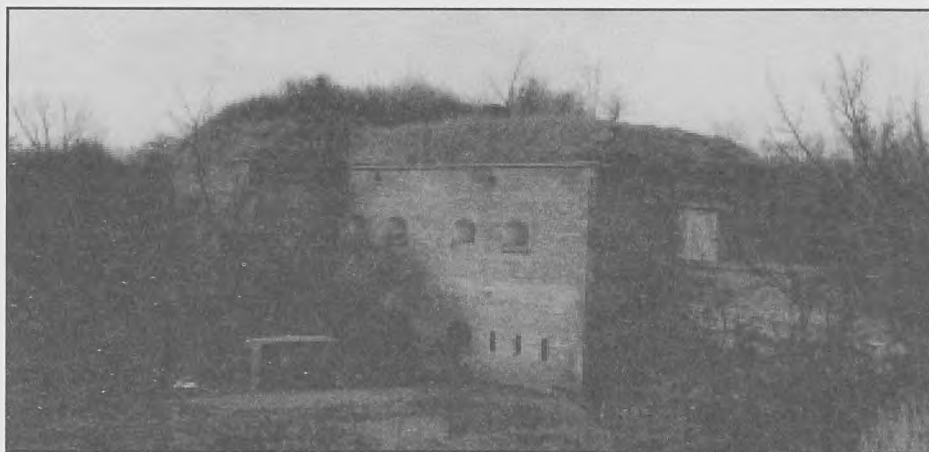
„Neoegipskie” kazamaty lunety przed Frontem Księcia Warszawskiego (obwód zewnętrzny)
