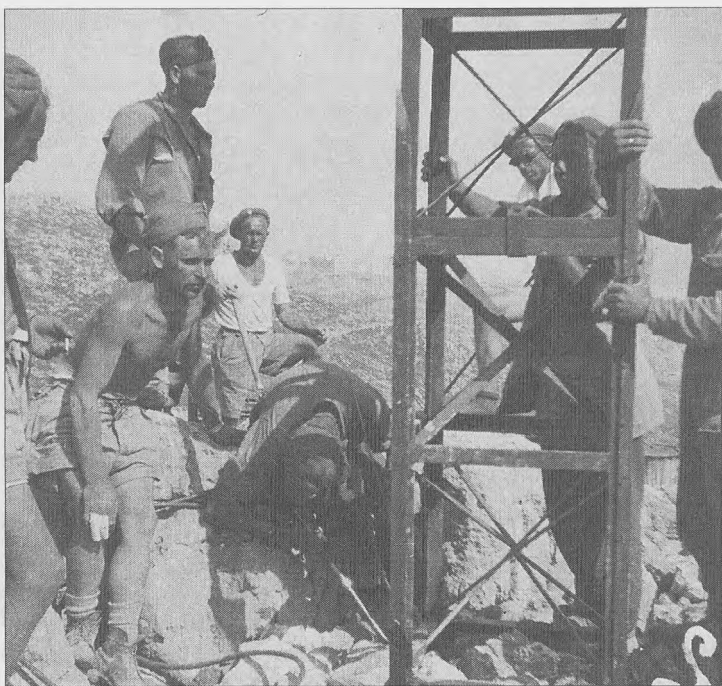
Fot. 36. Pionowanie konstrukcji. Za kratownicą stoi sap. Bolesław Abramczyk (z 14. KMK 2. BMK) i por. W. Kulikowski (w okularach)
