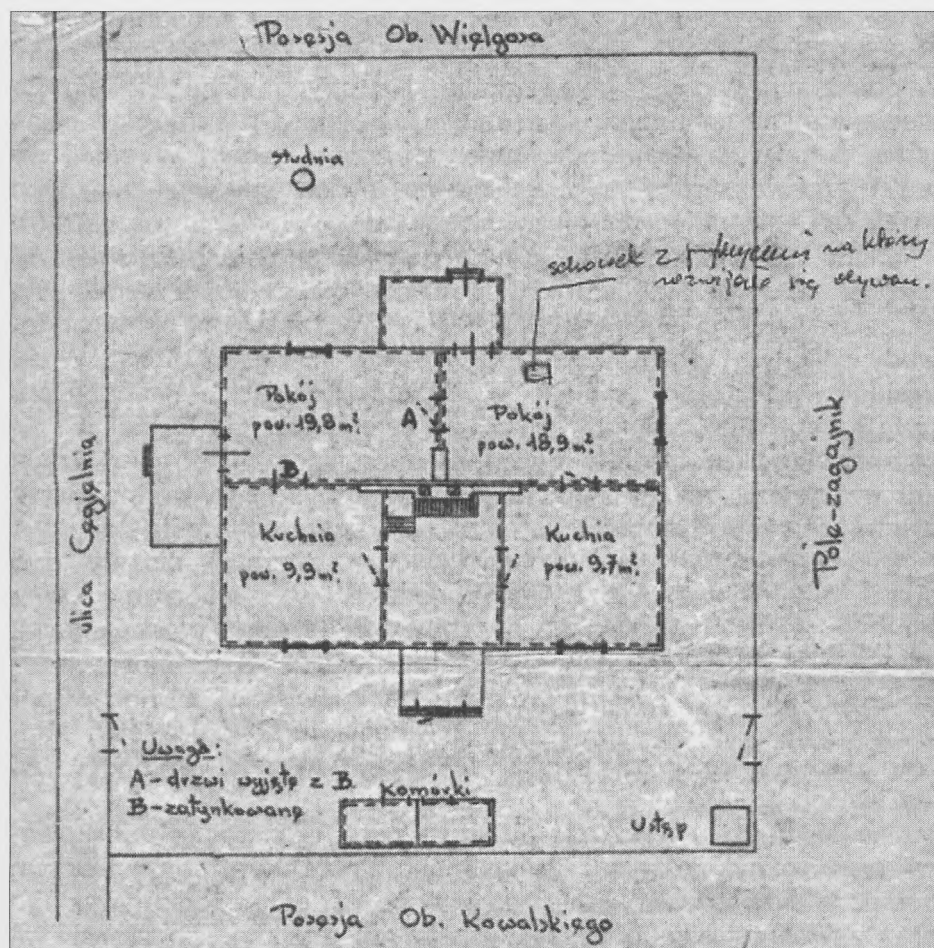
Fot. 6. Ogólny plan działki i parteru domu (oryginał znajduje się w Muzeum Historycznym w Legionowie)
