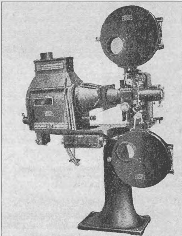
Fot. 5. Projektor Ernemann V. Projektor E IV konstrukcją nie różnił się zasadniczo od E V. Uproszczona w E IV była konstrukcja obiektywu i jego przesuwania, nie był chłodzony wodą. Miał pasowy napęd mechanizmu
