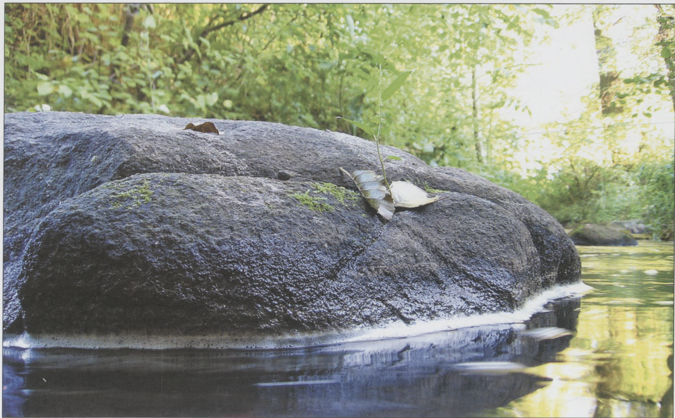
Głazy narzutowe w korycie rzeki przed Grodziskiem
